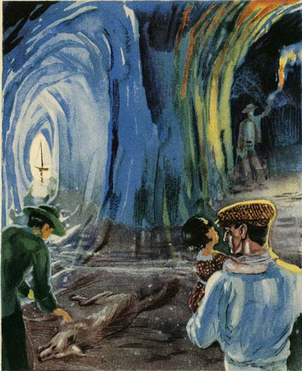
Bild 29: Die Hunde-Grotte auf der Insel Capri (Italien) In dieser Höhle lagert Kohlenäure über dem Boden. Hunde werden durch sie betäubt, aufrecht- stehende Menschen aber erreicht das Gas nicht
